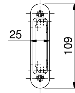
Art.nr.: 707023 Sluitkom
