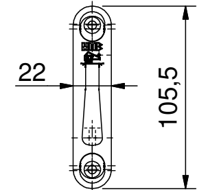
Art.nr.: 600357 Haakschootsluitplaat (inclusief 2 excenters)
